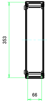
A-A (1:6.5)
